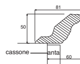
sezione cornice frame cross-section
